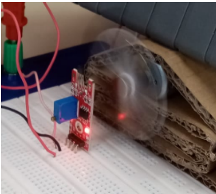
//Photo de gauche : capteur+MCC avec aimant - Photo de droite : carte NUCLEO-L476RG
